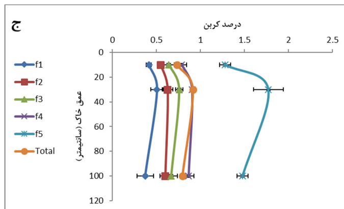
شکل ۵: نمودار توزیع کربن (± اشتباه معیار) در اجزاء اندازه‌ای خاک در اعماق مختلف منطقه شکار ممنوع (1000- 2000 μm, F2: 500- 1000 μm, F3: 250- 500μm, F4: 53- 250 μm, F5: <53 μm, کل خاک: Total)
